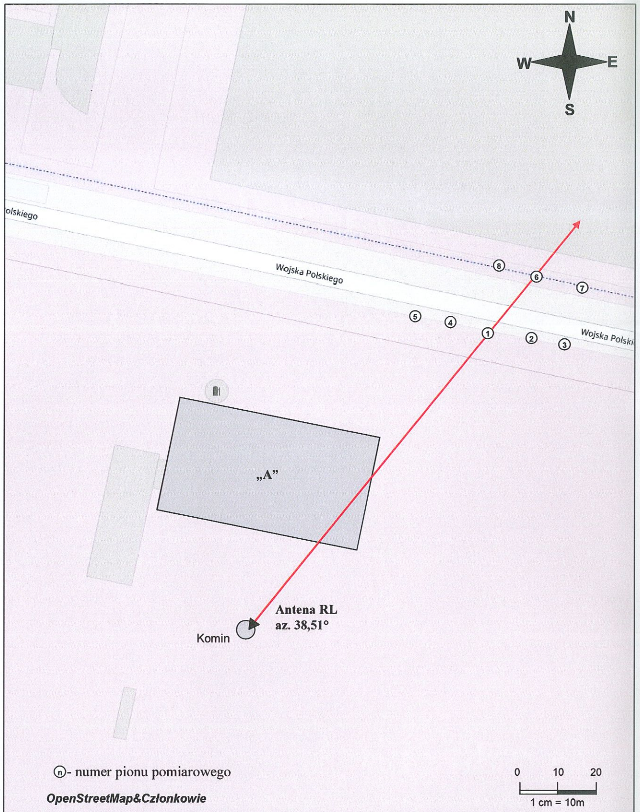
Rys. 1. Usytuowanie punktów i pionów pomiarowych w otoczeniu instalacji radiokomunikacyjnej Stacja Netia MIELB017-MIELM00002ANT003 Mielec, ul. Wojska Polskiego 3
