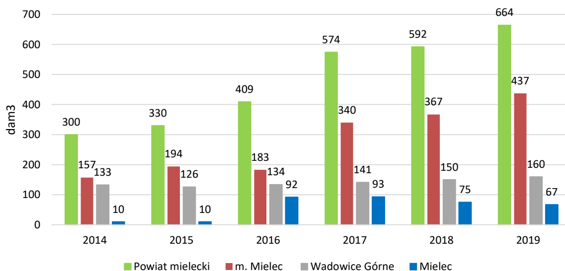
Rysunek 59. Zużycie wody na potrzeby przemysłu w powiecie mieleckim w latach 2014-2019
